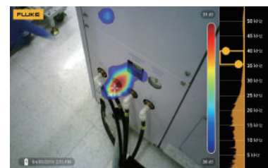
使用 Fluke ii900 進行氣體洩漏查找
