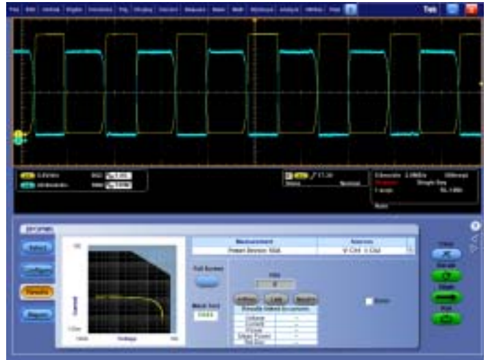
安全工作區量測，自動化功率量測能夠快速準確地分析常用功率參數。
