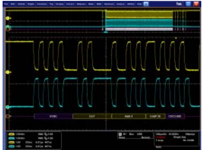
在一個全速的 USB 串列匯流排上觸發一個特定 OUT Token 封包。匯流排波形提供解碼封包內容，包含開始、同步、PID、位址、結束點、CRC、資料值和停止。
