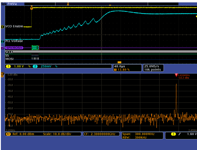
圖 3 — 頻譜時間再向右移動 120 \mu\text{s} 。在這個點上，頻譜顯示 PLL 實際上已超過正確的頻率，一直到 2.4164 GHz。
