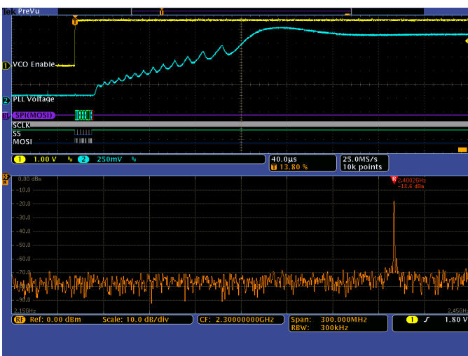
圖 4 — 約在 VCO 啟用後的 340 \mu\text{s} ，PLL 終於穩定在正確頻率 2.400 GHz 上。
