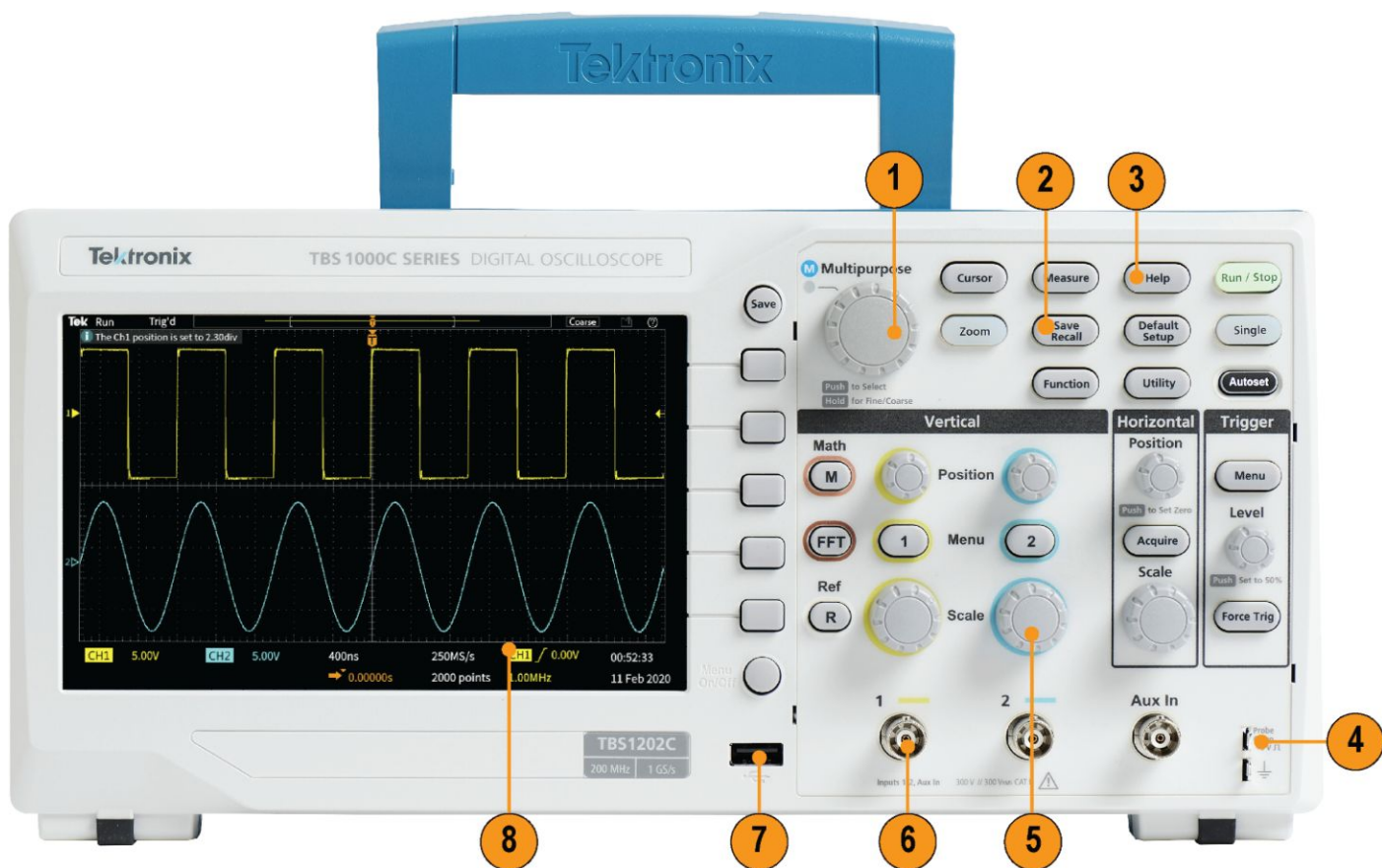
TBS1000C 前面板
