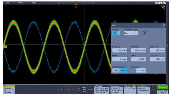
靈活的 AFG 輸出設定。在此測試案例中，20% 的雜訊已新增至正弦波形。
