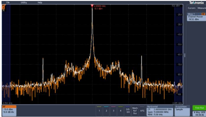
自動化通道電源量測
