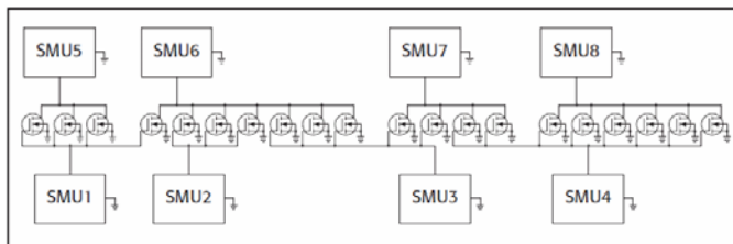
圖 7. 使用 8 個 SMU 來加壓並列的 20 個裝置以進行 HCl 和 NBTI 的範例。獨立的接地裝置 (GNDU) 用於公共終端。
