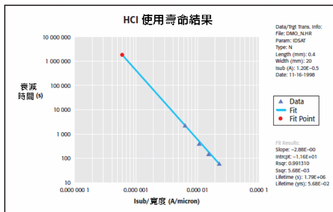
圖2. 從 HCI 測試壽命所作的可靠性推斷範例。
