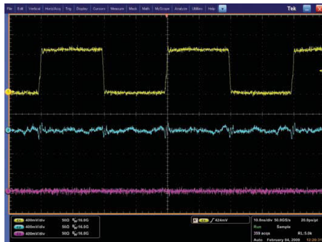
圖 42. 差動式探棒可以將目前快速低壓應用中的共模雜訊，與感興趣的訊號成分分開，這一點尤其重要，因為數位訊號正不斷下降到低於積體電路中典型雜訊臨界值的基準。
