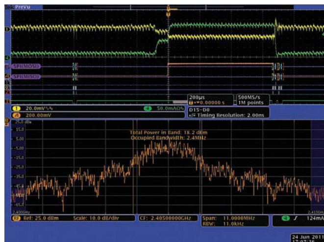
圖 16. Zigbee 無線電的微處理器 PI (MOSI) 和 (MISO) 控制線的時間相關顯示，量測到無線電 IC 的汲極電流和電壓及啓動期間的頻譜。
