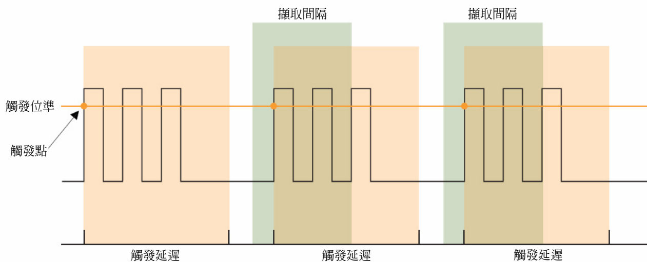
圖 36. 觸發延遲。
