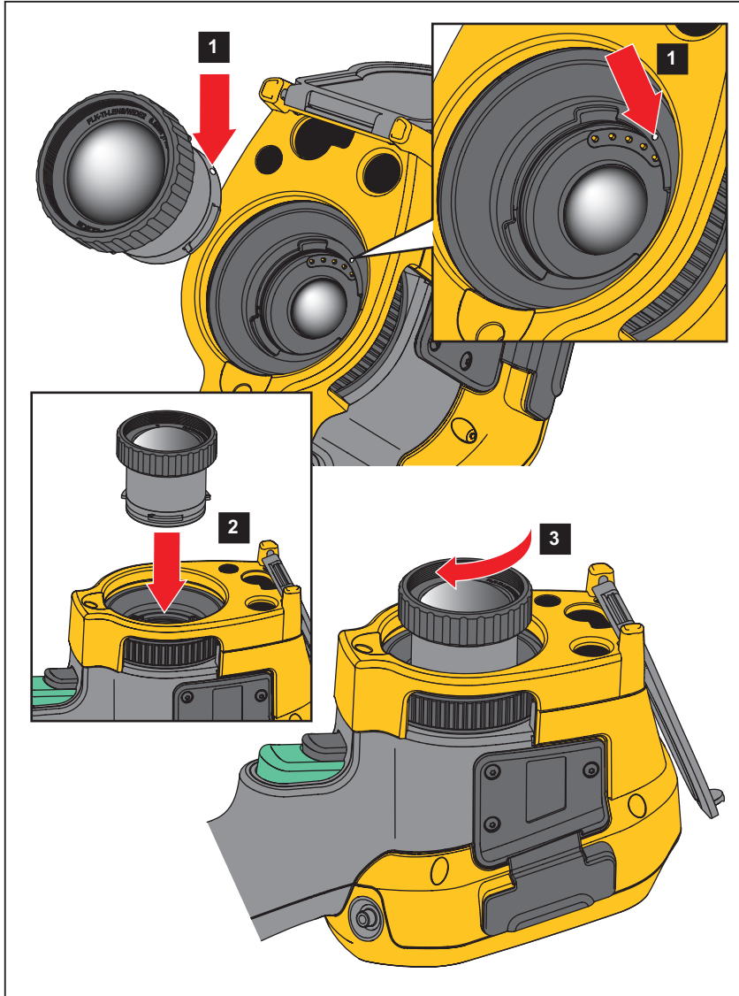
圖 2. 選用鏡頭的安裝
