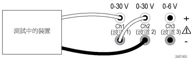
圖表 3: 機型 2230-30-1 和測試中裝置的串列設定。機型 2220-30-1 的串列設定是一樣的，但是通道 2 在最右邊。
