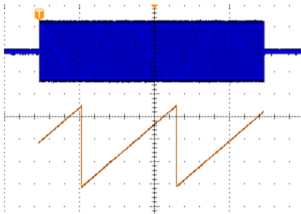
靜噪開啟
