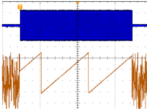
靜噪關閉
