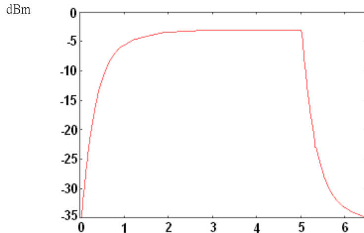
RF 功率偵測器回應 100 MHz 500 週期正弦波爆衝
